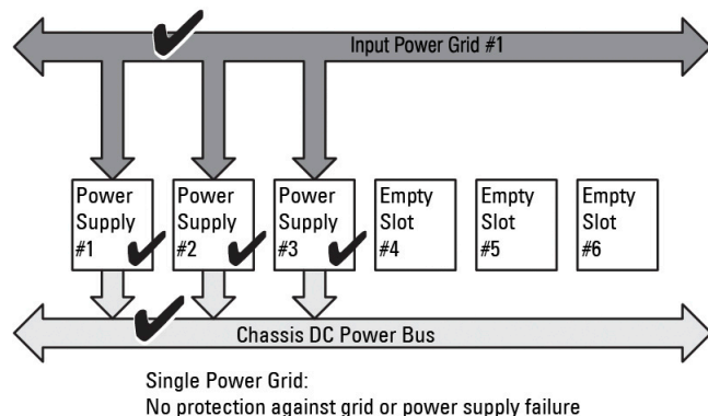
Figure 7. Mode Sans redondance avec trois blocs d'alimentation dans le châssis
